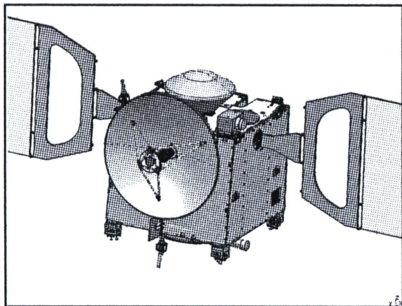
Esquema de la Mars Express, portadora de la perdida Beagle 2
